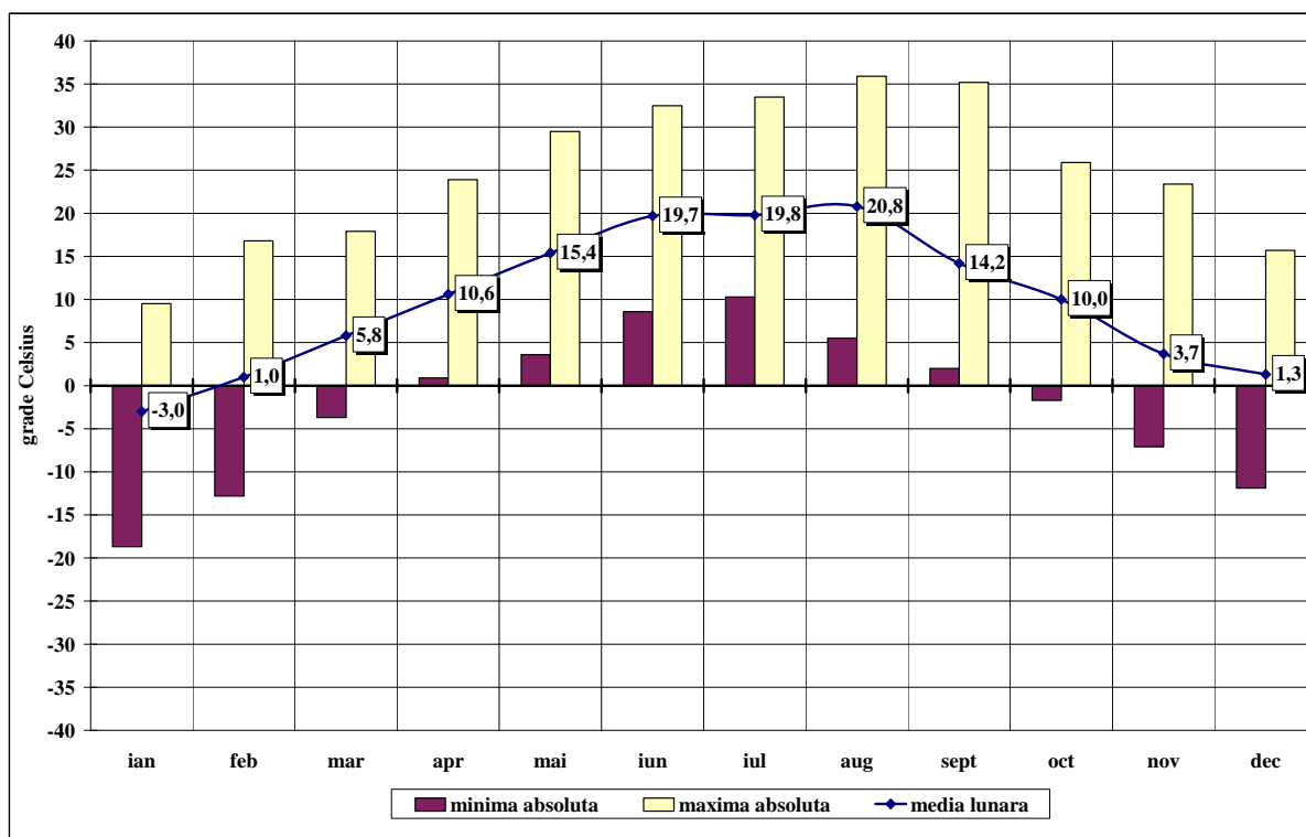
TEMPERATURA AERULUI - maxima absolută, minima absolută și media lunară - în anul 2008
